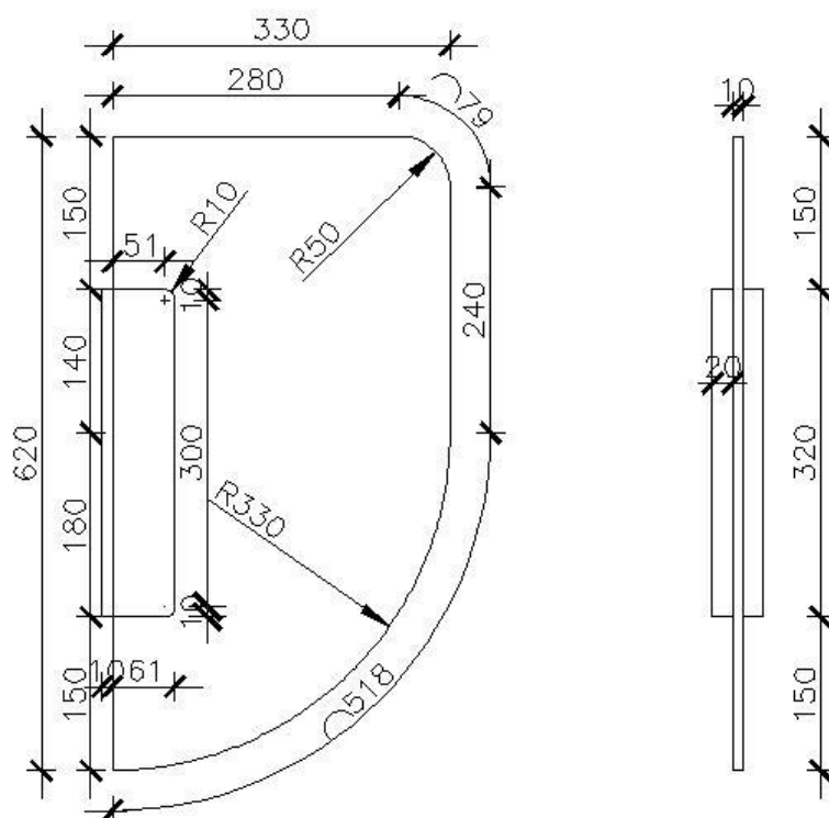
Rys.5.10.4. Wymiary projektowanej ścianki międzypisuarowej.
