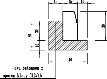
krawężnik betonowy 15x30x100cm
