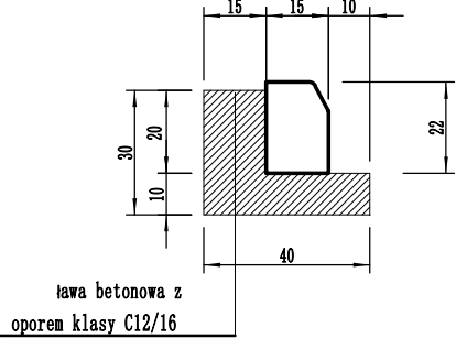
krawężnik najazdowy 15x22x100cm
