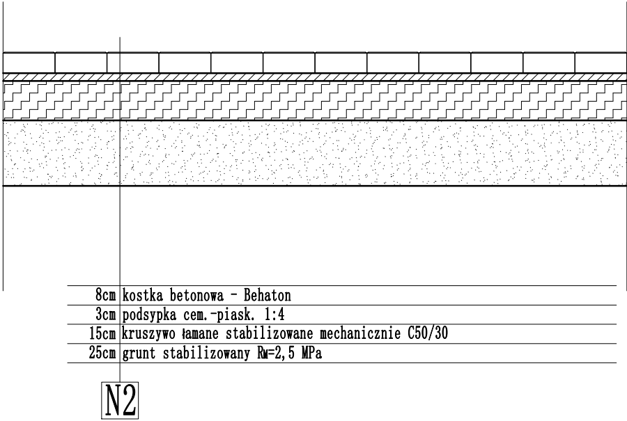
przekrój nawierzchni placu manewrowego dla samochodów osobowych
