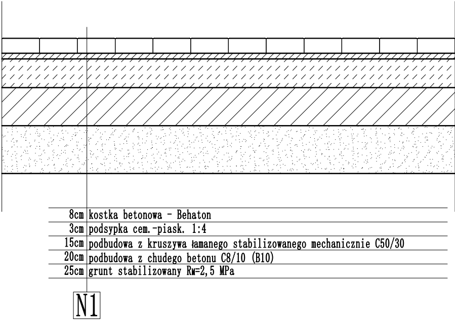
przekrój nawierzchni placu manewrowego dla samochodów ciężarowych
