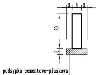
Obrzeże betonowe 8x30x100cm
