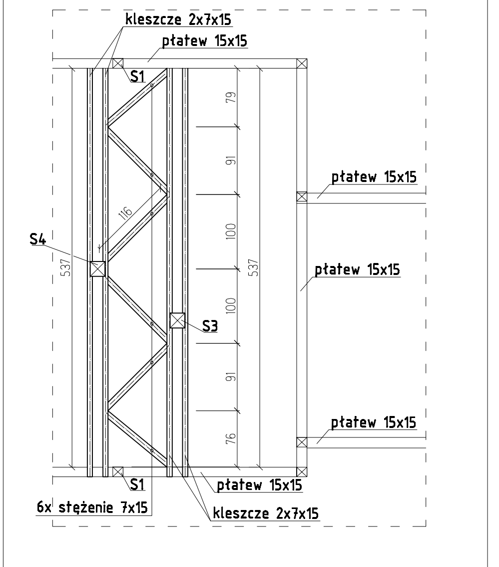
DETAL 2 Usztywnienie projektowanych słupów S3 i S4 - rzut na poziom płatwi
