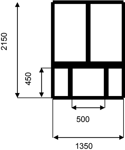
Przeszklenie z oknem podawczym 1 szt.
