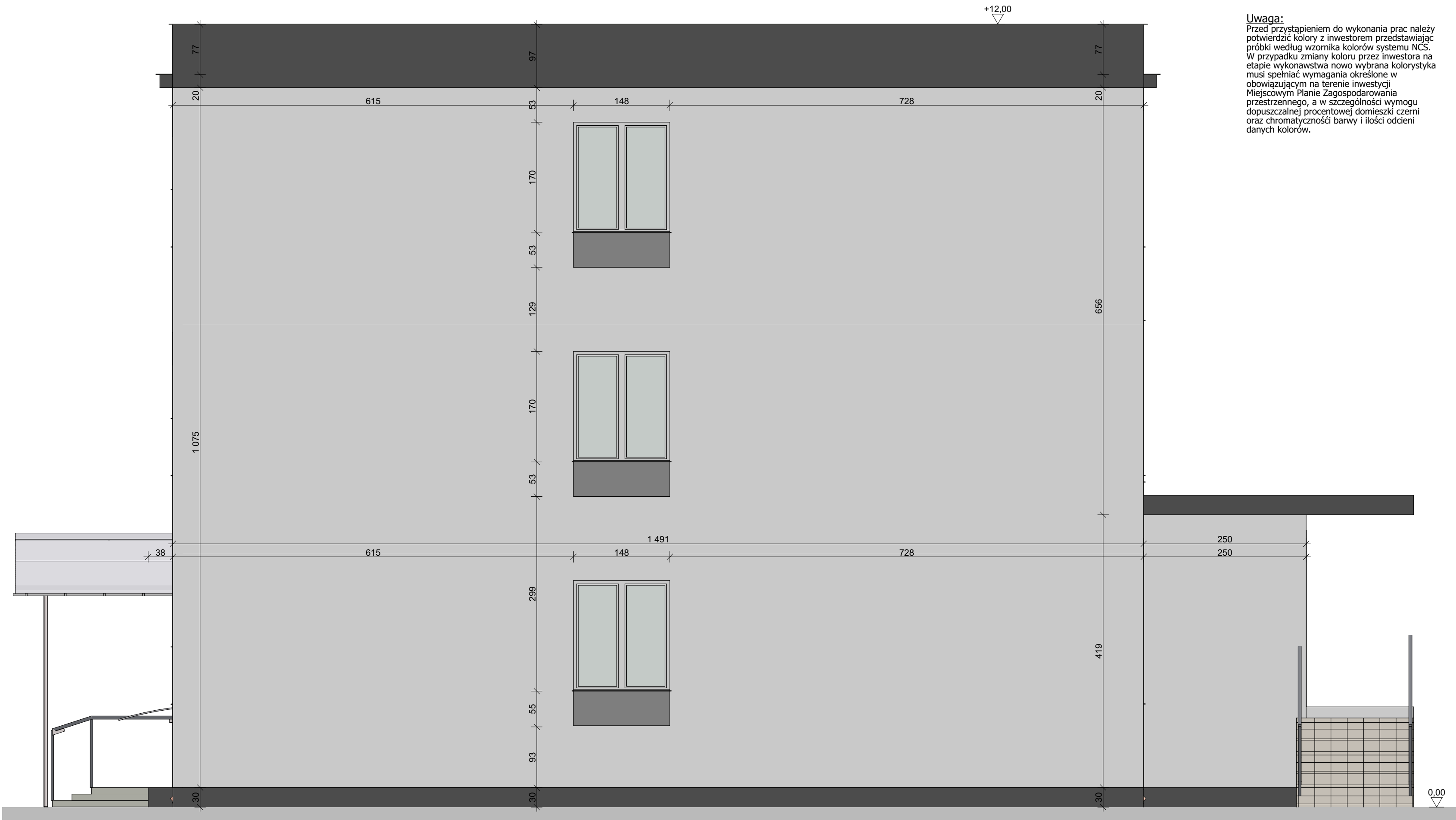
E-04 Elewacja południowa 1:50
