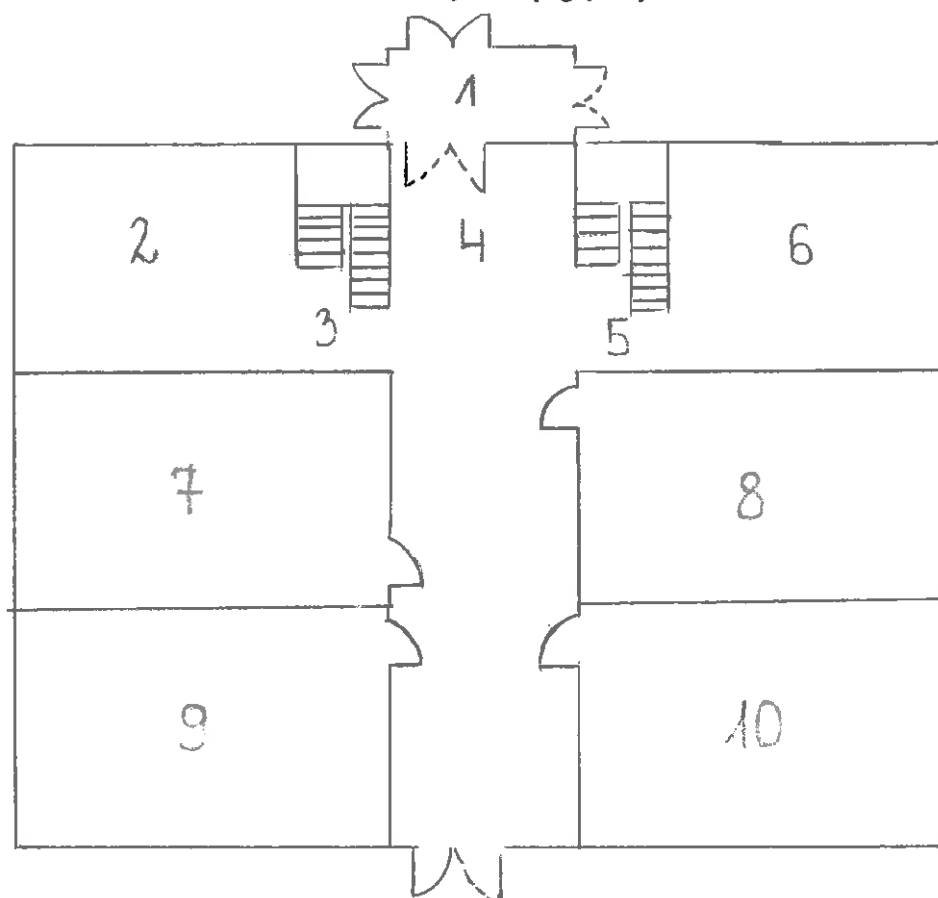
Rozkład pomieszczeń - parter Rysunek poglądowy
